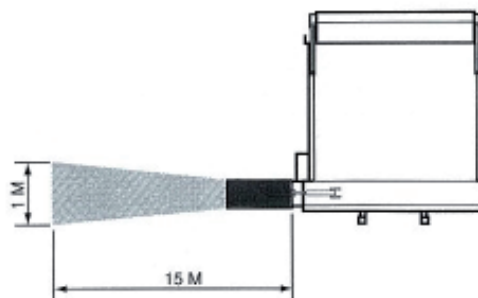
GOULOTTE STANDARD HAUTE
