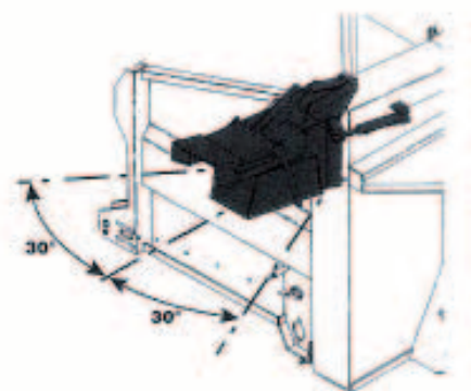
GOULOTTE ORIENTABLE + 30° AVANT / + 30° ARRIERE
