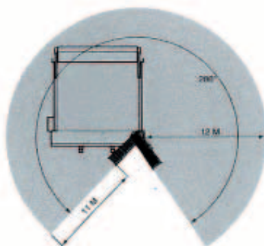
GOULOTTE ROTATIVE 280°
